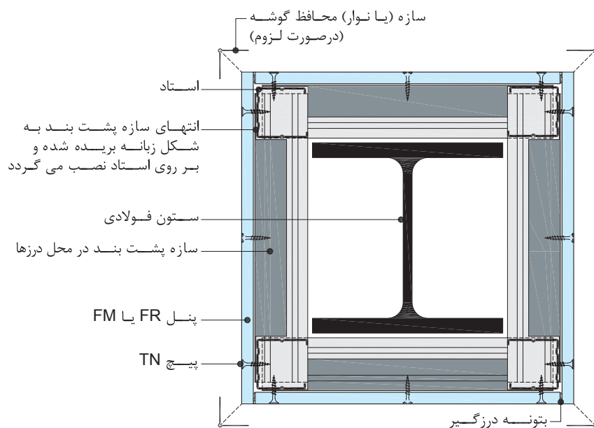
پوشش محافظ ستون - تک لایه (مقطع سازه‌های پشت‌تیر)
