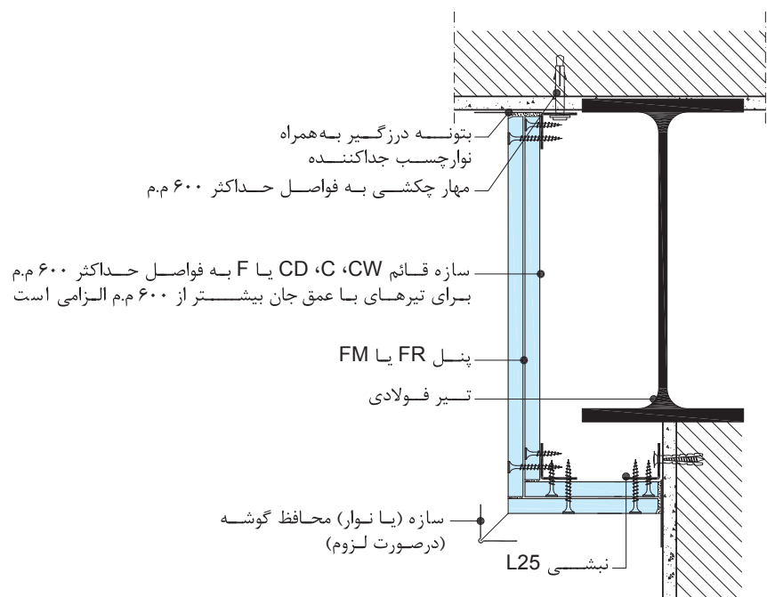
پوشش محافظ تیر گوشه
